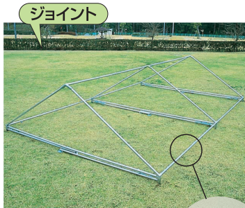
3つのパーツをおこし桁棟パイプを差し込みます。(※桁パイプは、差し込みを深くしているので天幕をかぶせれば抜けることはありません)
